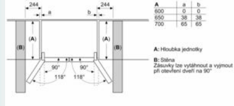
Rozměry v mm
